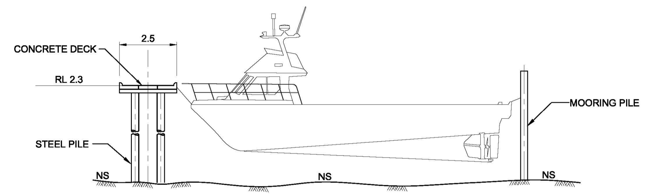
SECTION B-B Scale: 1 : 100
